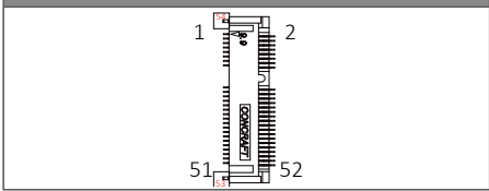
Mini PCIe Connector
