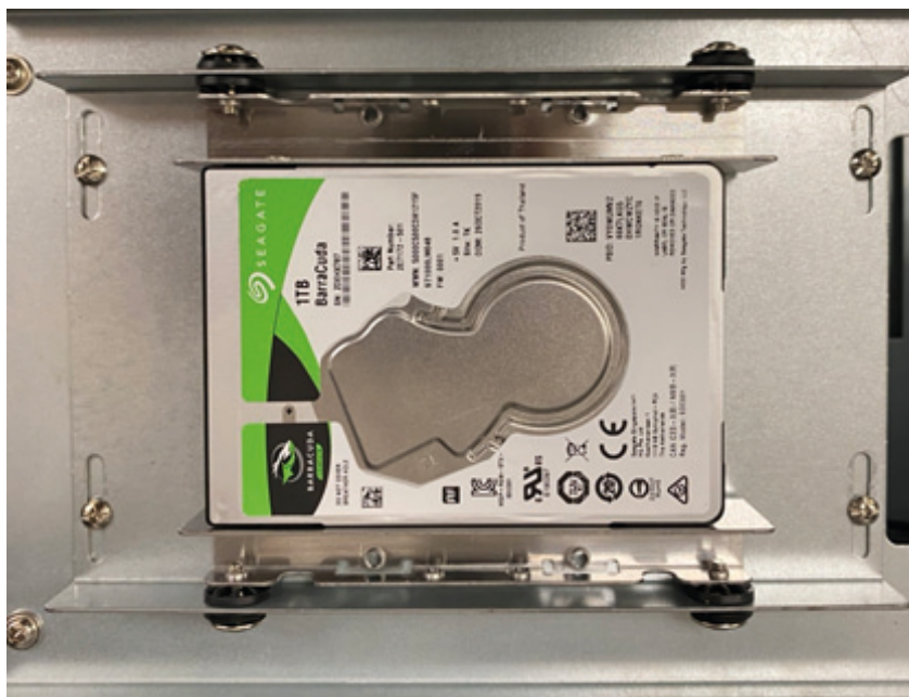
Figure 2.16 Installing HDDs and bracket with chassis/ 安裝硬盘与支架于机箱上 / 安裝硬碟與支架於機箱上
