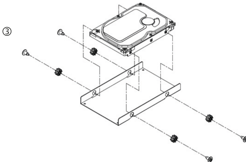
Figure 2.17 Installing second 3.5" HDD/ 安裝第 2 个 3.5" 硬盘 / 安裝第 2 個 3.5" 硬碟
