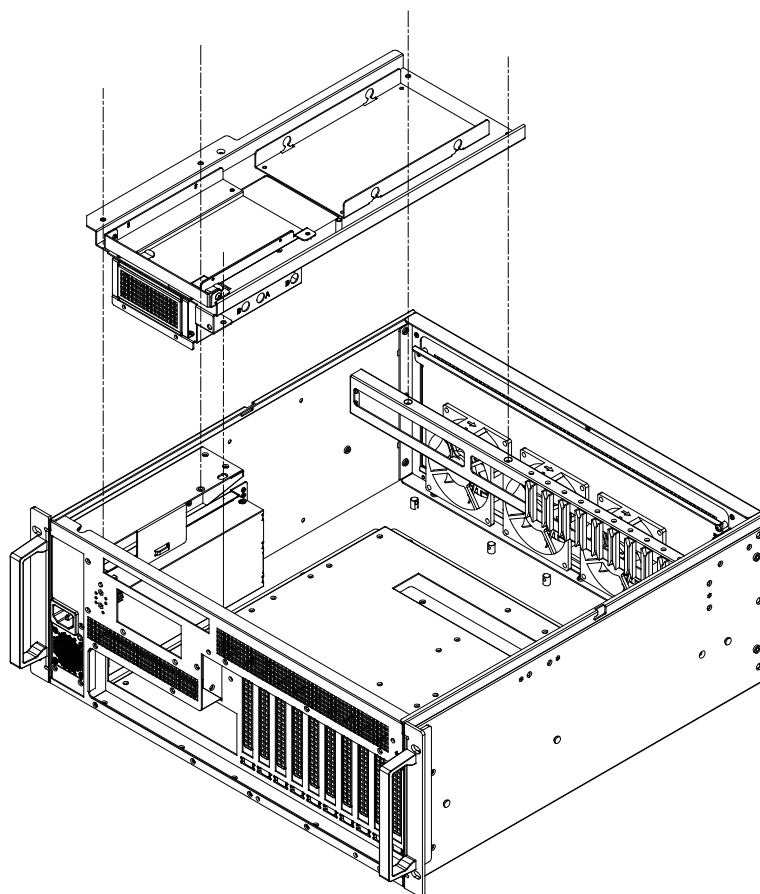
Figure 2.5 Remove second layer mechanism/ 移除层架式结构 / 移除層架式結構
