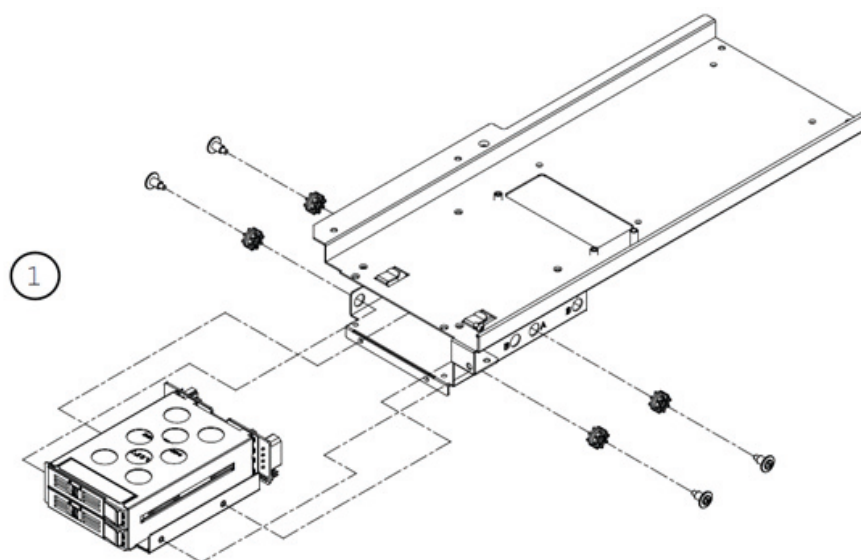
Figure 2.8 Installing two 2.5" external HDD trays/ 安装 2 个 2.5" 前置硬盘模块 / 安裝 2 個 2.5" 前置硬碟模組
