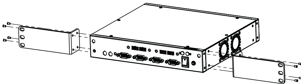
Figure B.3 Installing the Rack Mounting Bracket / 安装机箱 Rack 导轨安装支架 / 安装机箱 Rack 导轨安装支架
