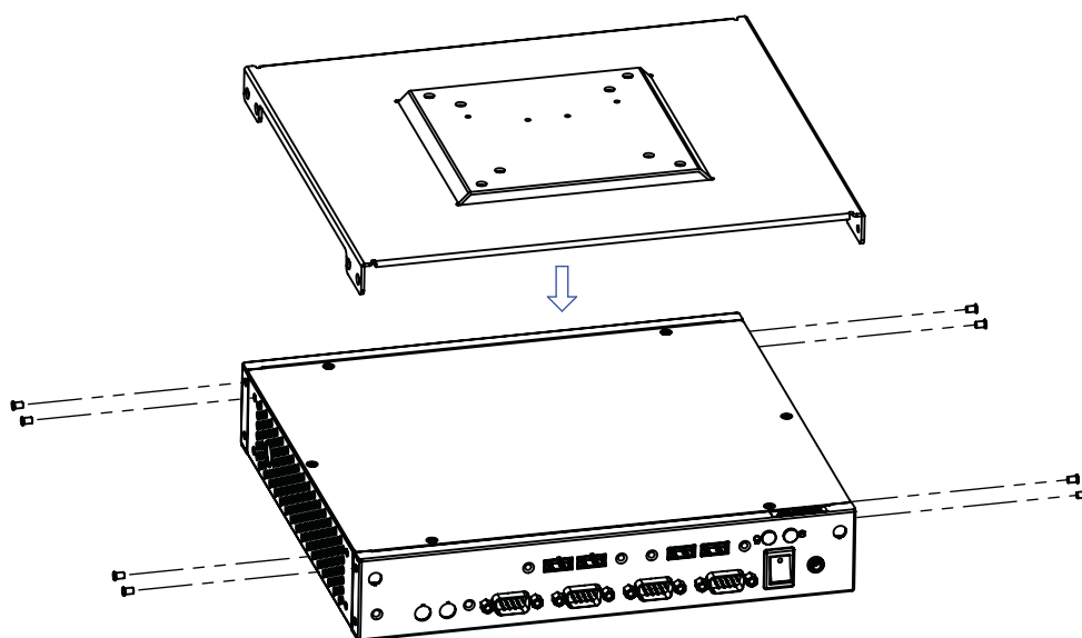
Figure B.2 Installing the VESA Mounting Brackets / 安装机箱底座 VESA 安装支架 / 安装机箱底座 VESA 安装支架
