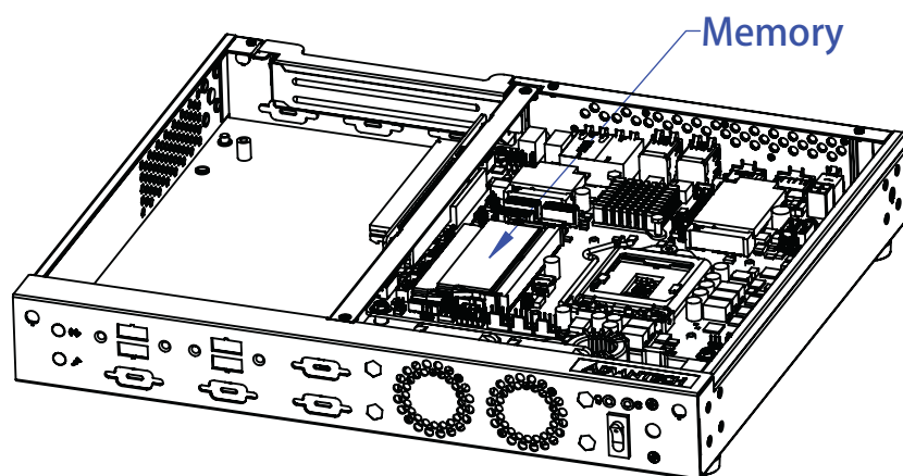
Figure 2.6 Installing the memory/ 安裝內存 / 安裝記憶體
