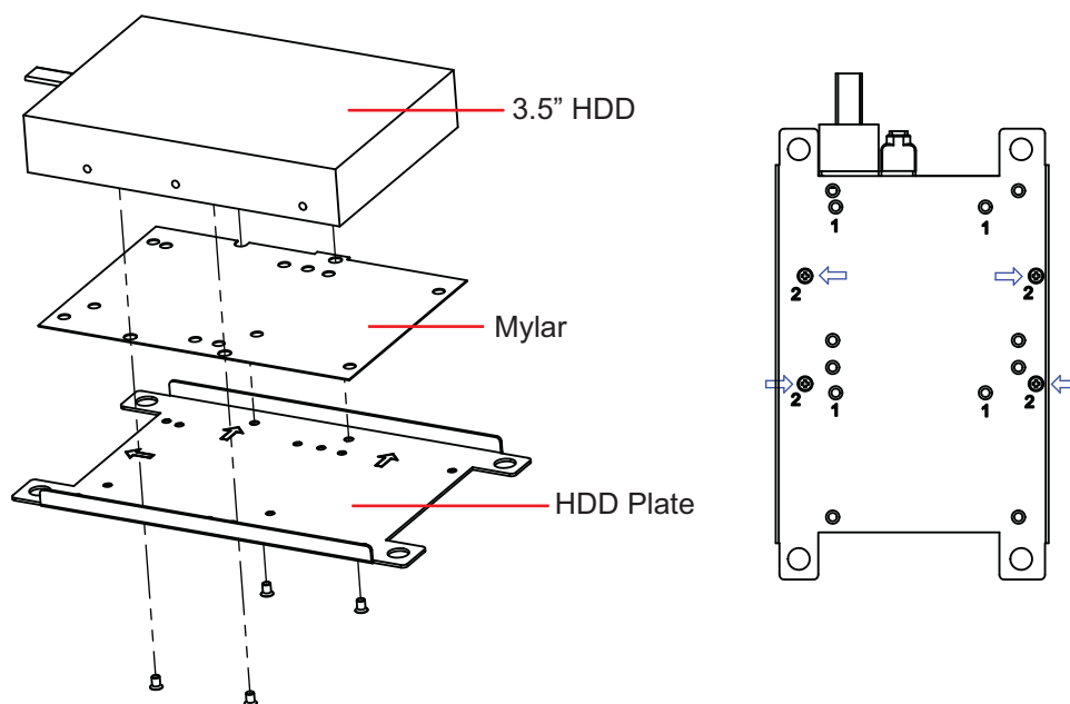
Figure 2.3 Assemble 3.5" HDD/SSD (vertical) / 組裝 3.5" 硬盘 (直式) / 組裝 3.5" 硬碟 (直式)
