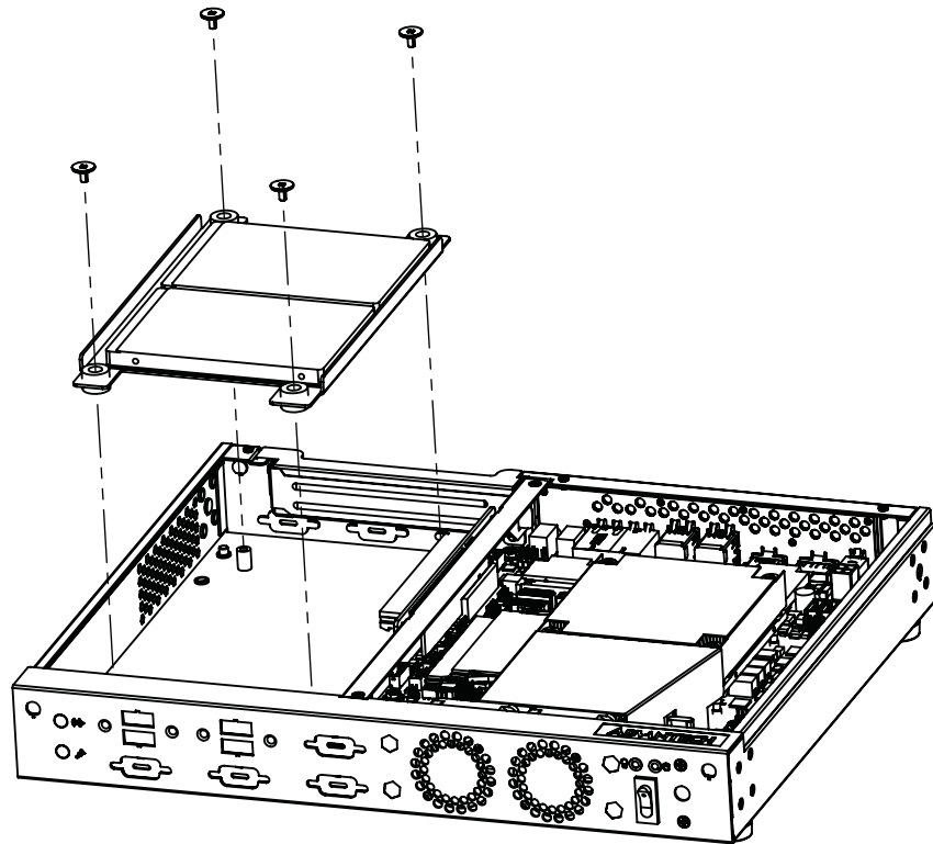
Figure 2.5 Assemble HDD and HDD bracket / 安裝硬盤与硬盤架 / 安裝硬碟與硬碟架
