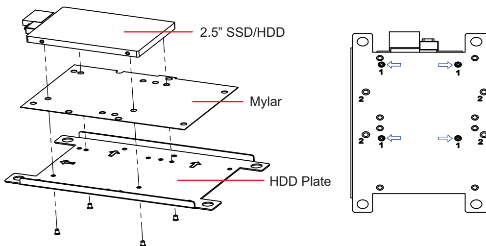
Figure 2.2 Assemble 2.5" HDD/SSD (vertical) / 组装 2.5" 硬盘（直式） / 組裝 2.5" 硬碟（直式）
