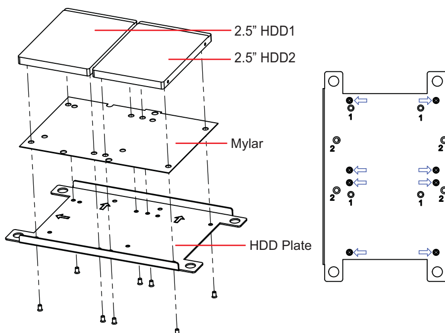
Figure 2.4 Assemble 2 x 2.5" HDD/SSD / 組裝 2 x 2.5" 硬盘 (橫式) / 2 x 2.5" 硬碟 (橫式)
