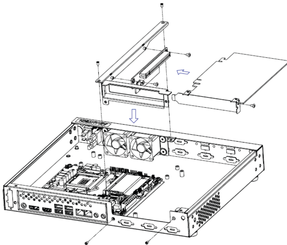
Figure 2.7 Installing & Changing PCIe x4 module/ 安裝和更換 PCIe x4 模块 / 安裝和更換 PCIe x4 模塊
