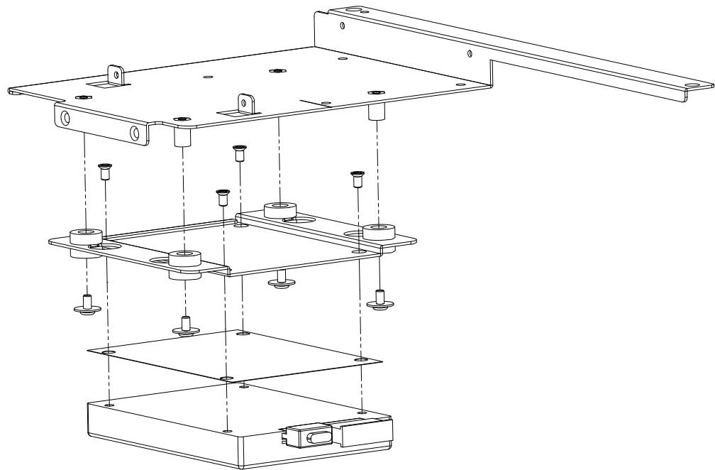
Figure 2.4 Installing HDD-2/ 安裝 HDD-2/ 安裝 HDD-2
