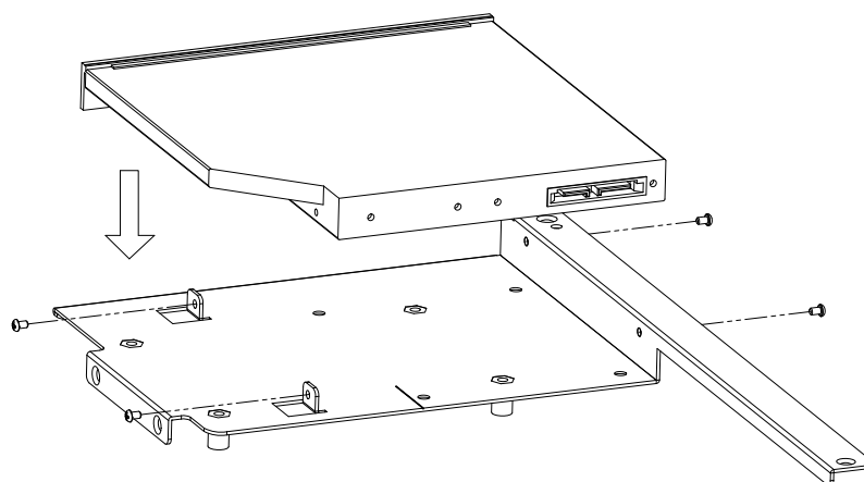
Figure 2.5 Install ODD / 安裝 ODD/ 安裝 ODD
