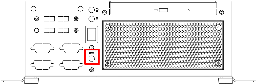
Figure 3.2 Reset button/ 电源重置按钮 / 電源重置按鈕
