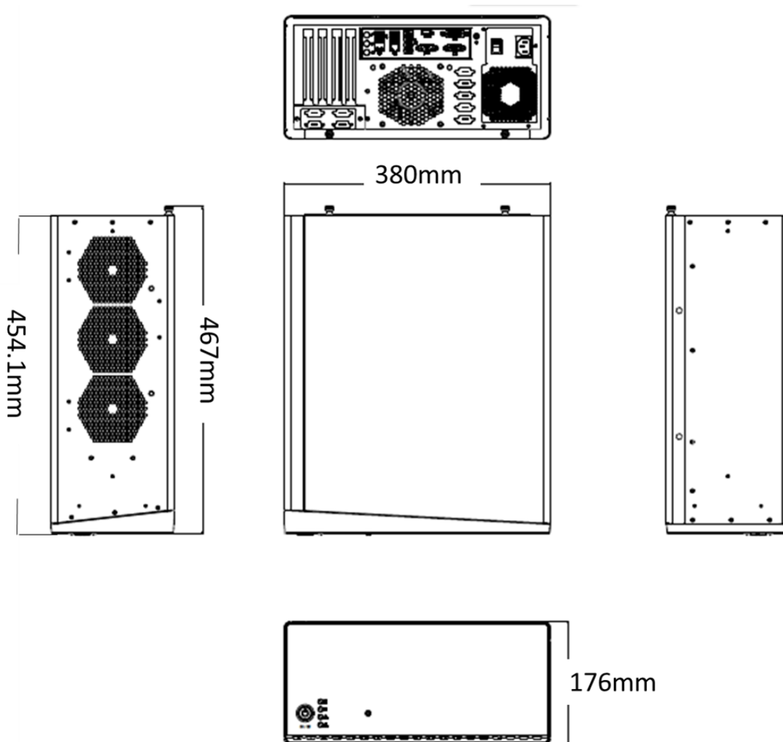
Figure 1.1 Dimensions/ 产品尺寸 / 產品尺寸
