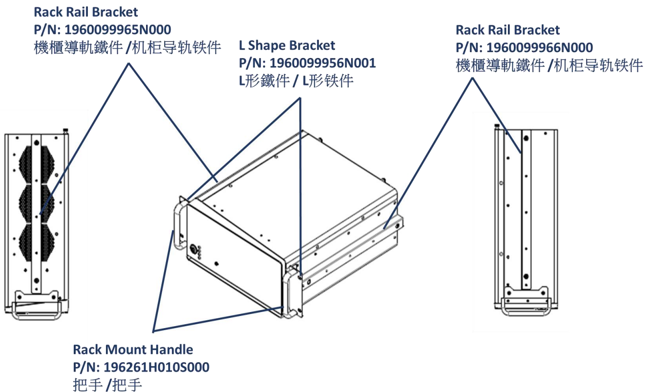
Figure 2.4.2 Installing Rack Mounting Bracket / 安装机箱 Rack 导轨安装支架 / 安裝機箱 Rack 導軌安
