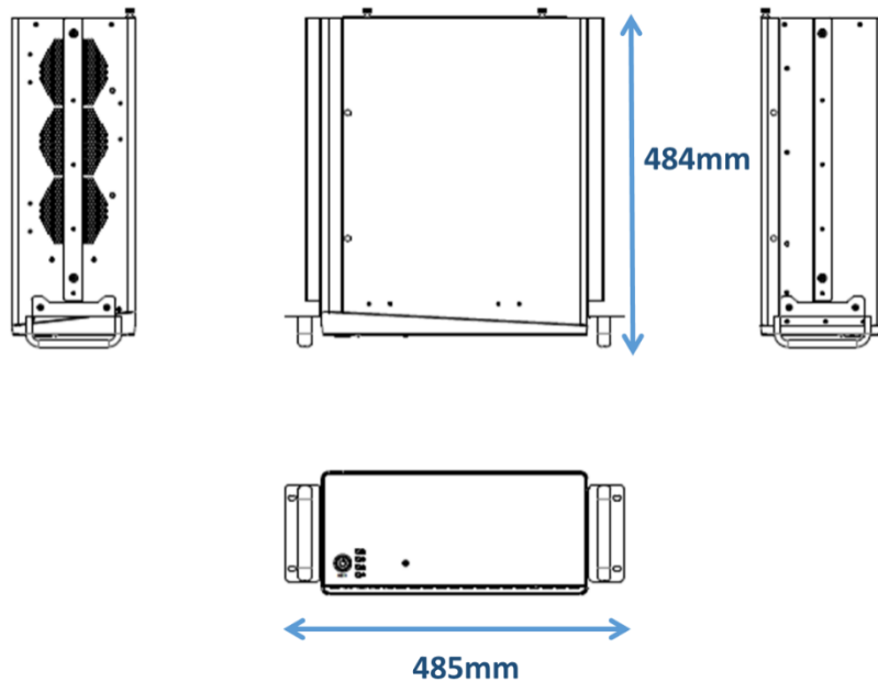
Figure 2.4.1 Installing Rack Mounting Bracket / 安装机箱 Rack 导轨安装支架 / 安裝機箱 Rack 導軌安裝支架
