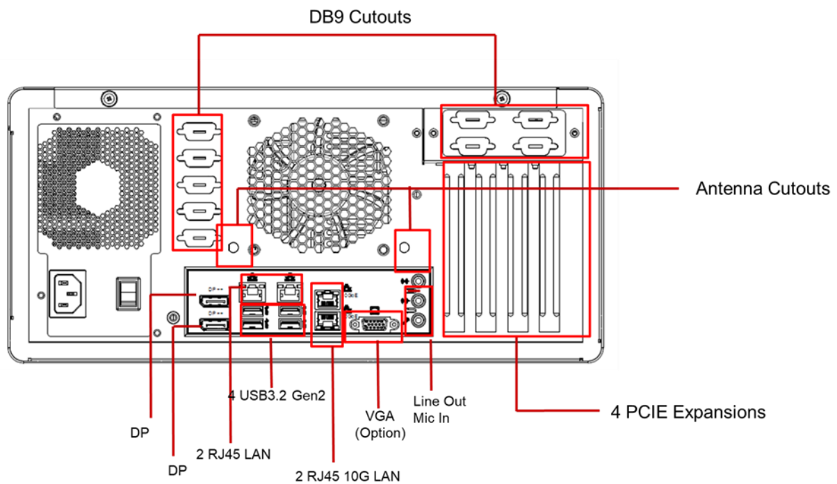
Figure 1.3 Rear View Diagram/ 产品后视图 / 產品後視圖
