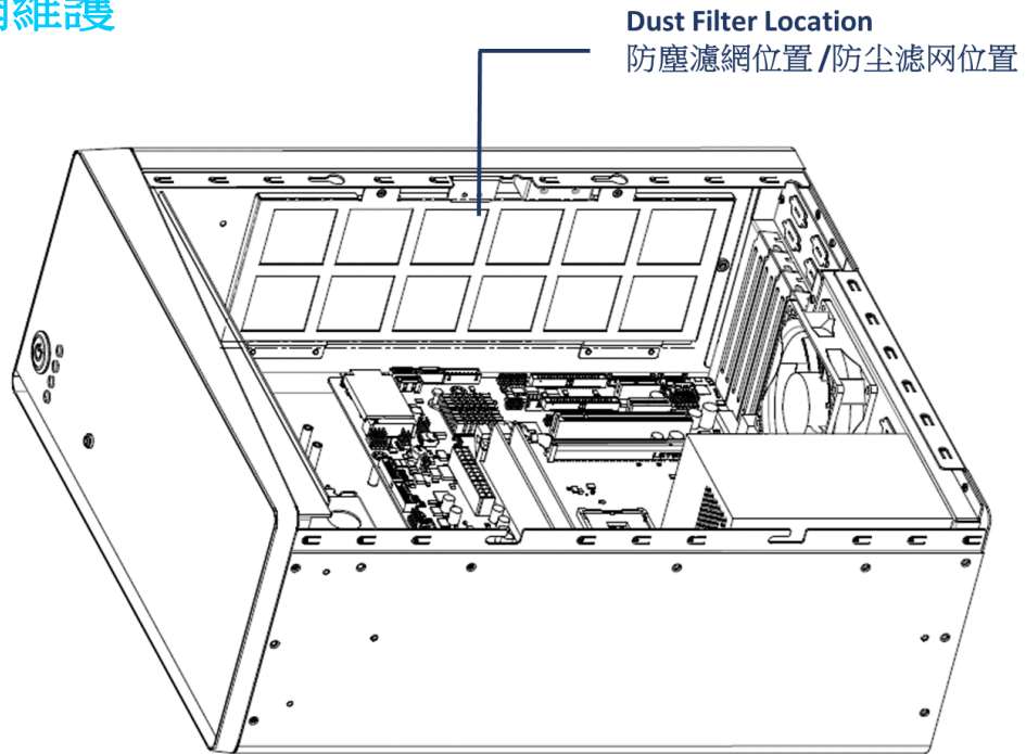
Figure 2.3.1 Dust-proof Filter Location / 防尘滤网位置 / 防尘滤网位置
