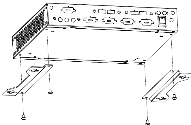
Figure B.1 Installing the Wall Mounting Brackets / 安装机箱底座壁挂式支架 / 安裝機箱底座壁掛式支架
