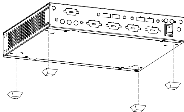
Figure 2.11 Installing Rubber Foot on Bottom Side/ 安裝机箱底部橡胶脚垫 / 安裝機箱底部橡膠腳墊
