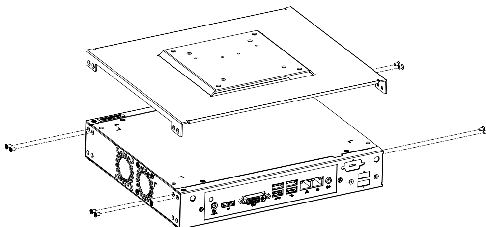
Figure B.2 Installing the VESA Mounting Brackets / 安装机箱底座 VESA 安装支架 / 安裝機箱底座 VESA 安装支架
