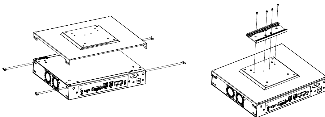
Figure B.3 Installing the DIN Rail Mounting Bracket / 安裝機箱底座 DIN 导轨安装支架 / 安裝機箱底座 DIN 導軌安裝支架
