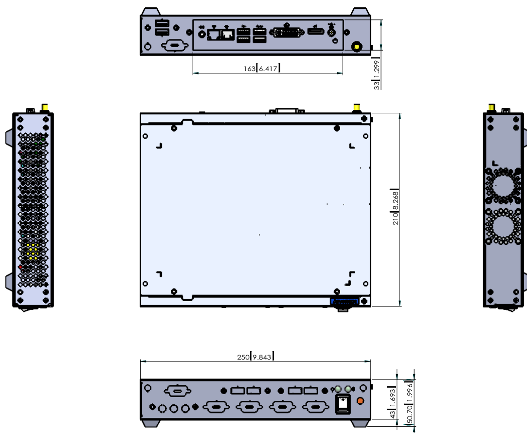
Figure 1.1 Dimensions/ 产品尺寸 / 產品尺寸
