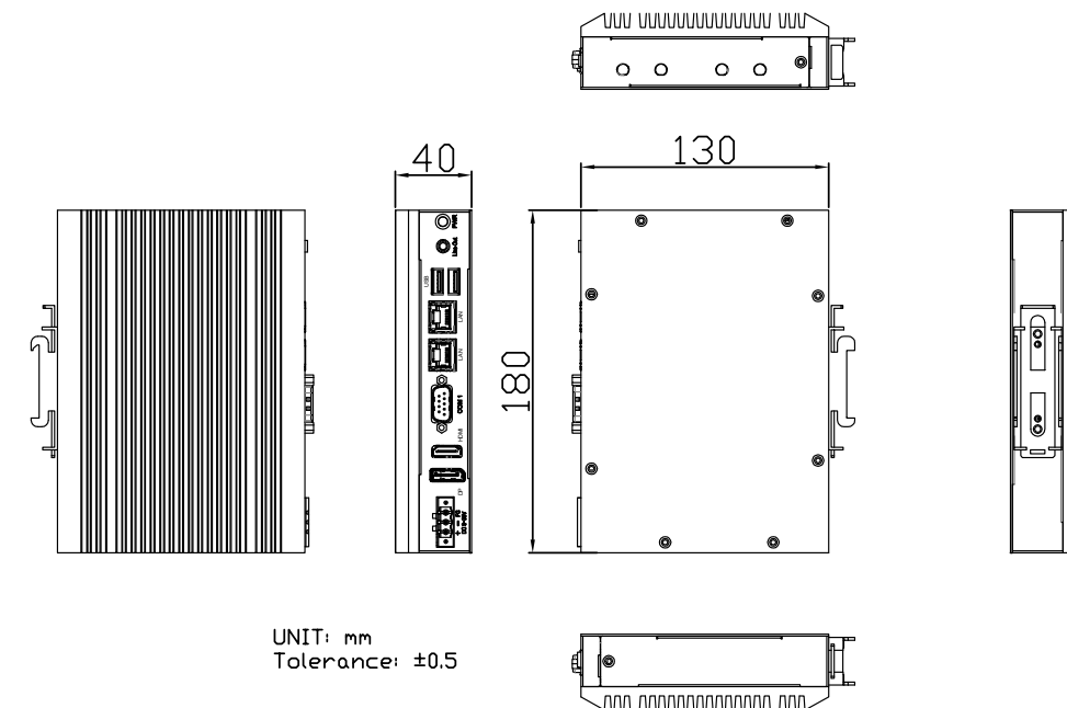
ACS-2310A DIN Rail
