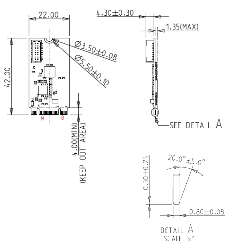
EGP2-X204-W1 (Vertical Connector)
