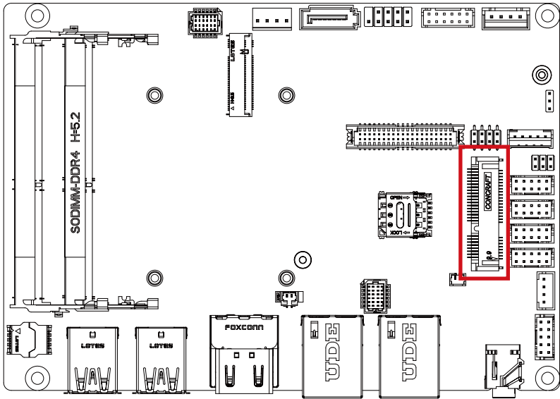
Mini PCIe Connector
