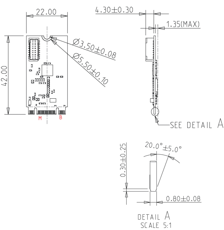
EGP2-X203-W1 (Vertical Connector)
