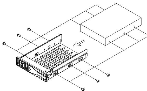
Figure 2.8 Installing a SATA HDD/ 安装 SATA 硬盘 / 安裝 SATA 硬碟
