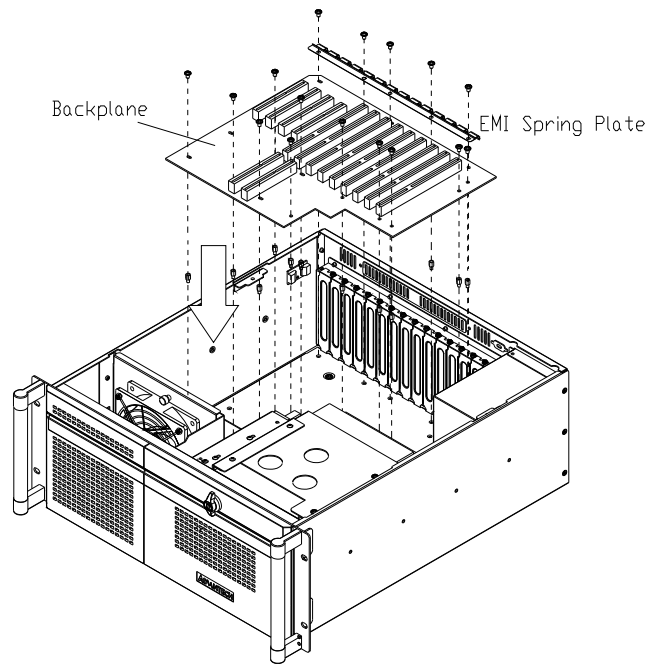
Figure 2.3 Installing the Backplane/ 安装底板 / 安装背板
