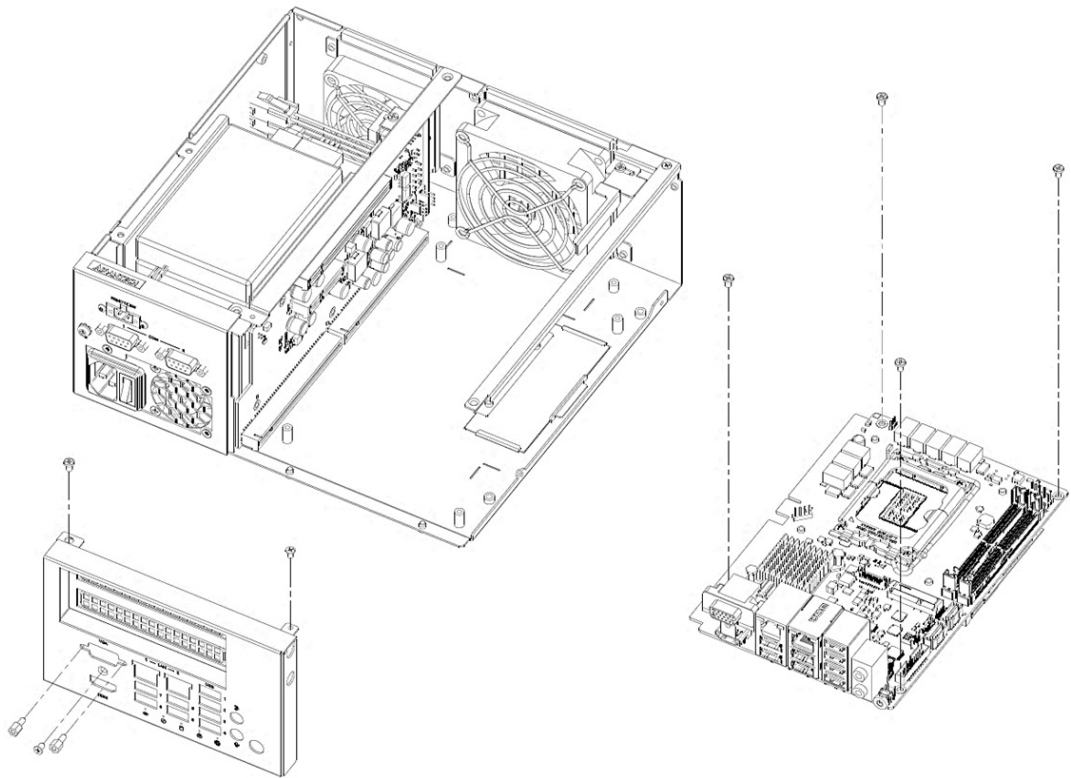
Figure 2.1 2.1Installing CPU Board / 安裝 CPU 板 / 安裝 CPU 板
