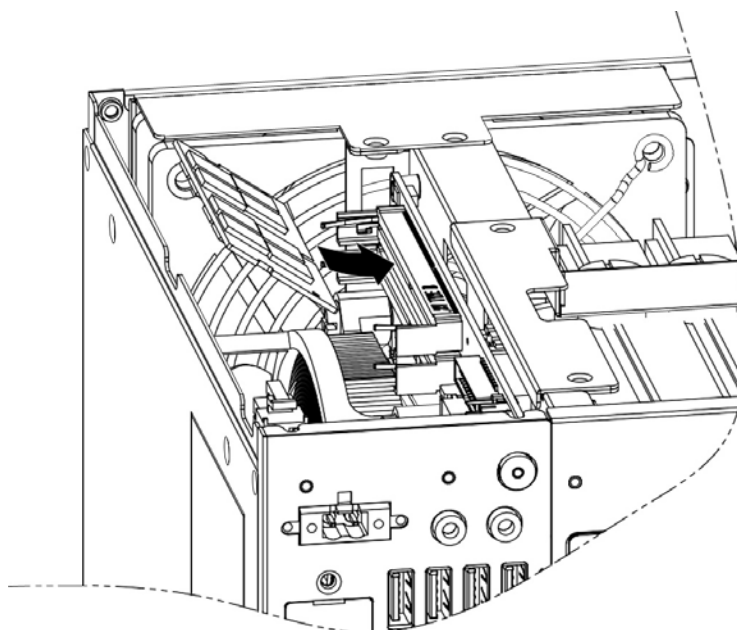
Figure 2.4 Memory Installation / 内存安装 / 記憶體安裝
