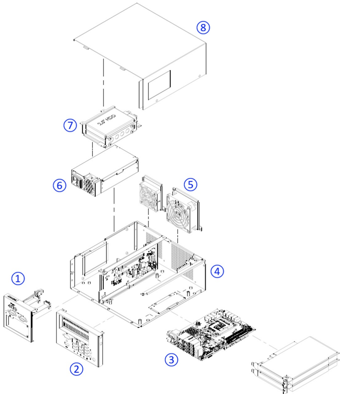
Figure A.1 Exploded Diagram / 分解图 / 分解圖
