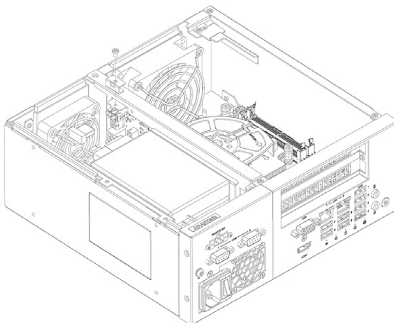
Figure 2.5 Internal USB dongle installation / 内部 U 盘安装 / 内部 USB 安装
