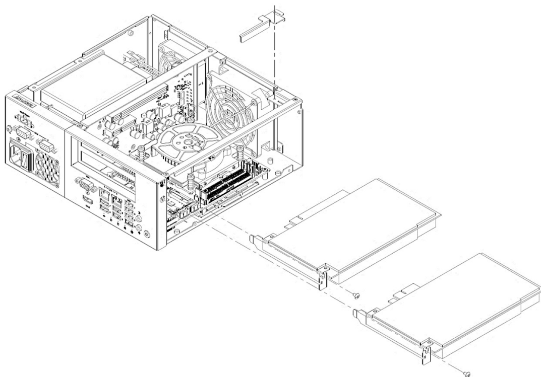
Figure 2.3 Installing Add-On-Card / 安装扩展卡 / 安裝擴充卡
