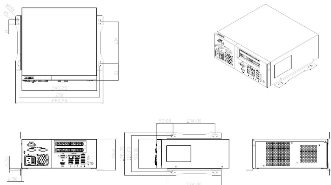
Figure 1.1 Dimensions / 产品尺寸 / 產品尺寸
