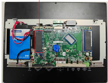
貼附 M.2 Thermal pad
